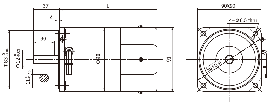
图11 90YS60 ( 60W ) 交流三相电机, 长度L=123mm ) ;
